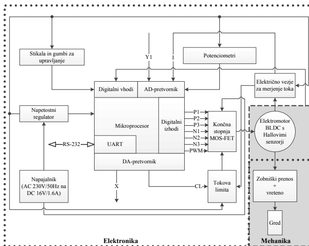
Slika 2: Shematski prikaz električnih vezij in komponent povezanih z mehanskimi deli pogona.
