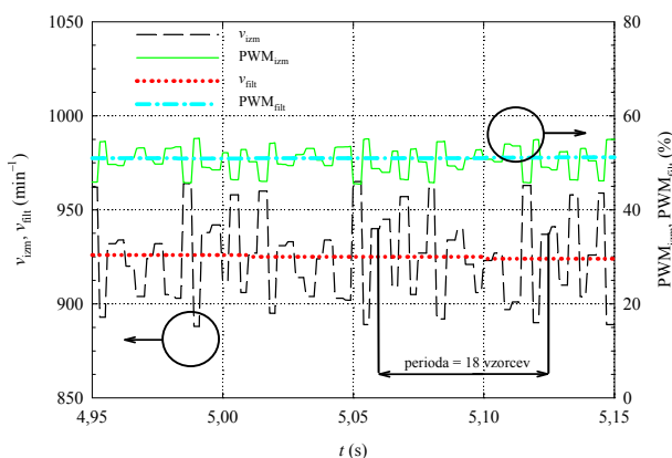
Slika 10: Izmerjena ( v_{izm} ) in filtrirana hitrost ( v_{filt} ) s pripadajočim razmerjem PWM_{izm} in PWM_{filt} kot funkcija časa t v ustaljenem stanju.
